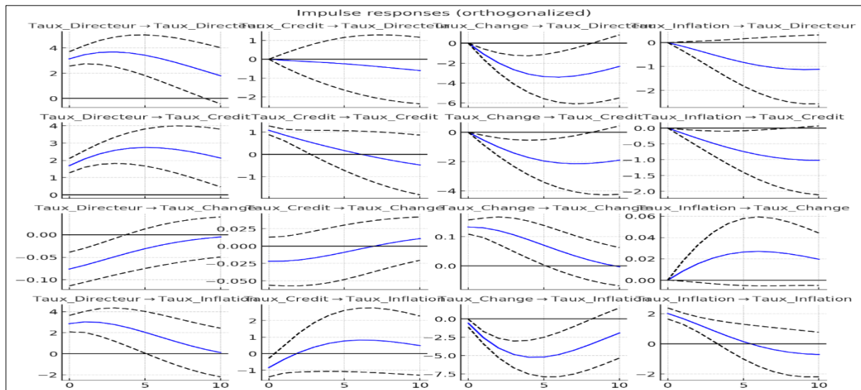
Figure 1. Réponses impulsionnelles orthogonalisées issues de VAR
